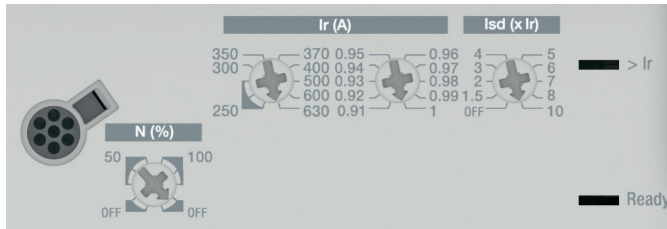
Trip unit LSnI
