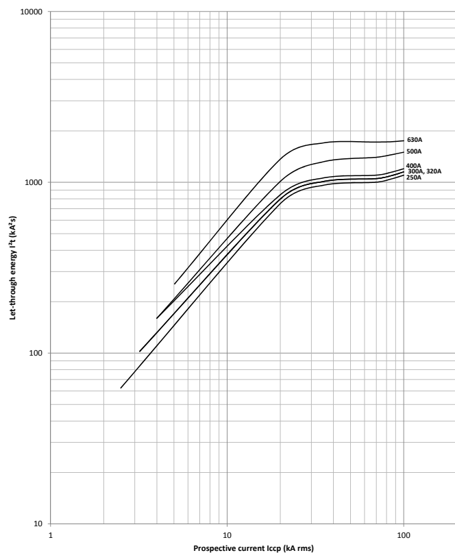
x630 TM
